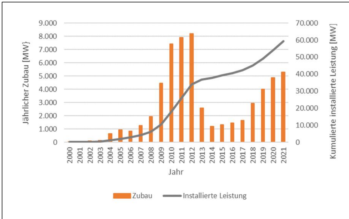
Abb. 2.2: Installierte Leistung und Zubau an PV-Anlagen von 2000 bis 2021
